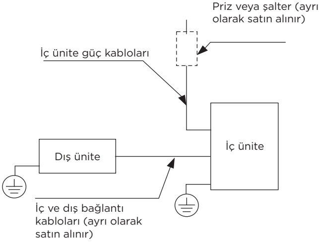
İç mekan güç kaynağı modelleri
