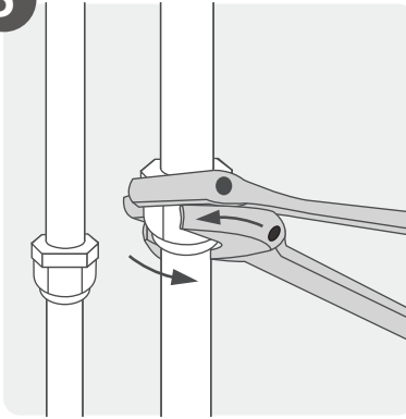
Boruları Bağlayın
