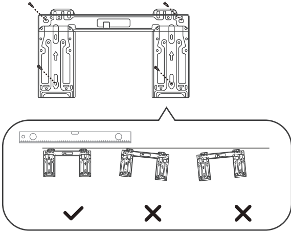
Montaj Plakasının doęru yönlendirilmesi
