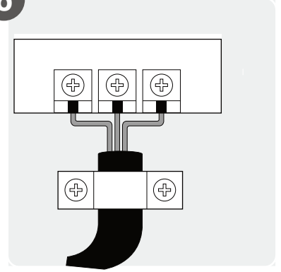
Kabloları Bağlayın
