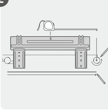
Montaj Plakasını Takın
